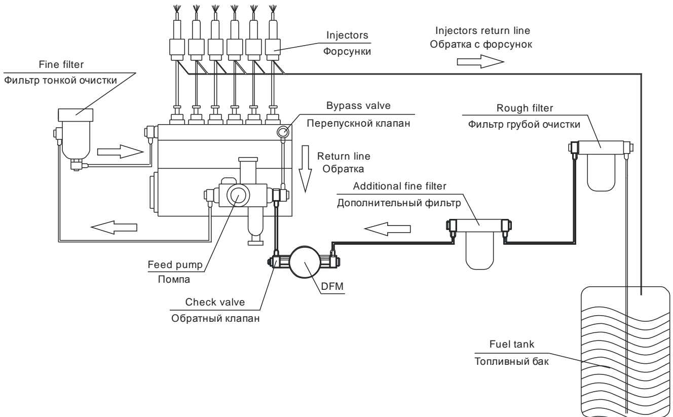
Рис. 2 Установка DFM на разрежение
