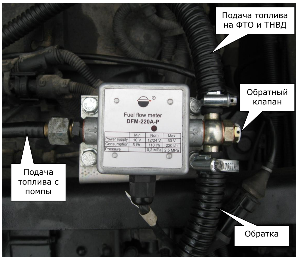
Рис. 8 Объединение подачи топлива и обратки на выходе DFM
