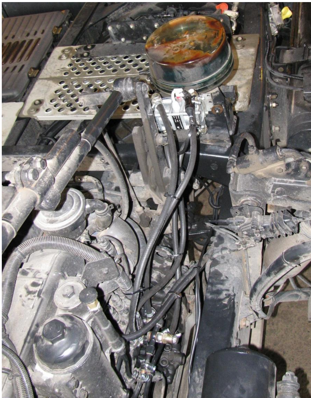
Рис. 10 Установка DFM по дифференциальной схеме на двигателе MAN
