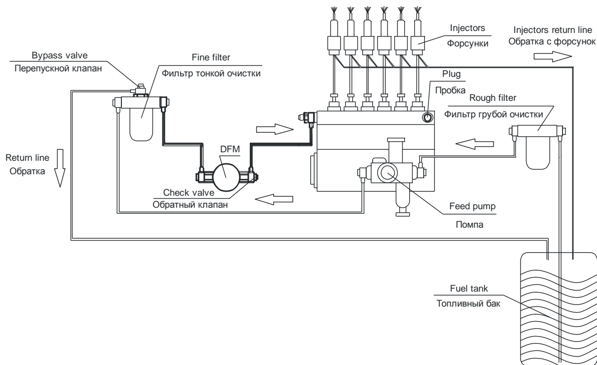
Рис. 3 Установка DFM на давление
