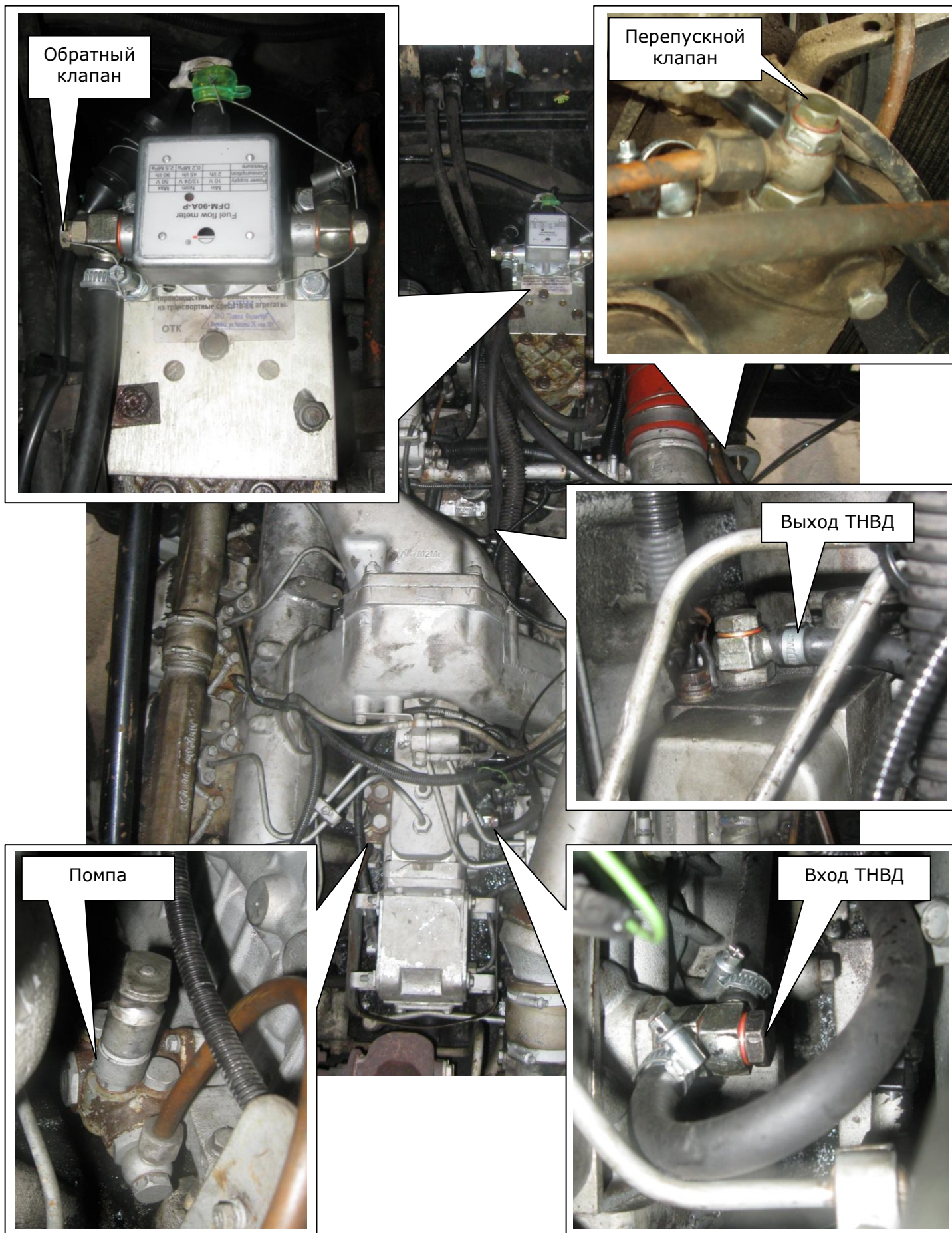
Рис. 5 Установка DFM по схеме на давление
