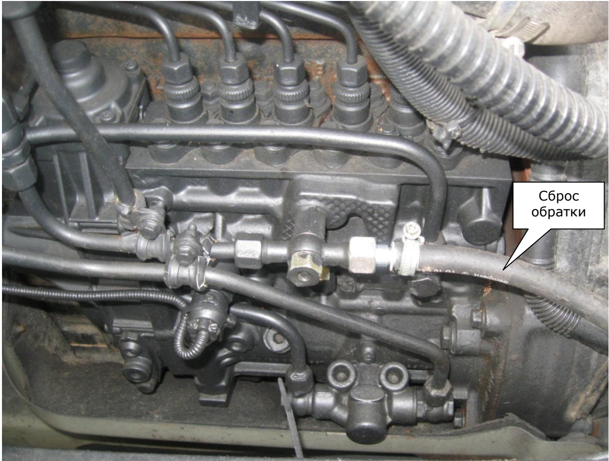
Рис. 7 Обратка с фильтра тонкой очистки и ТНВД
