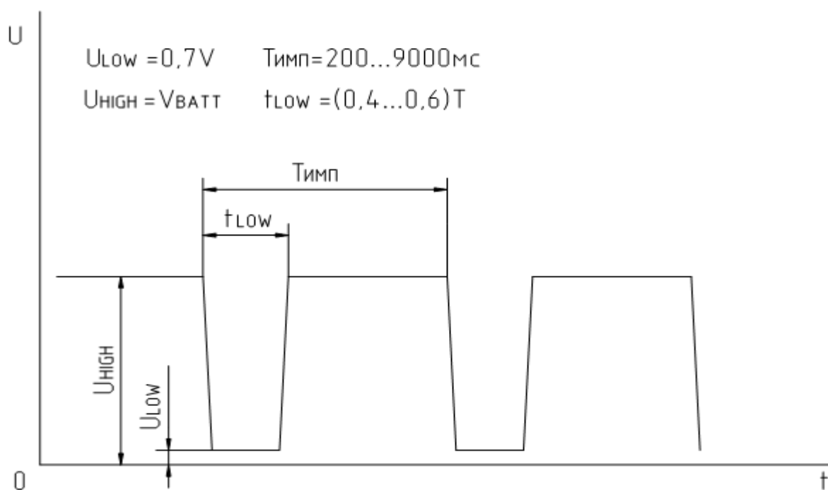
Рис. 1 Выходной сигнал DFM
